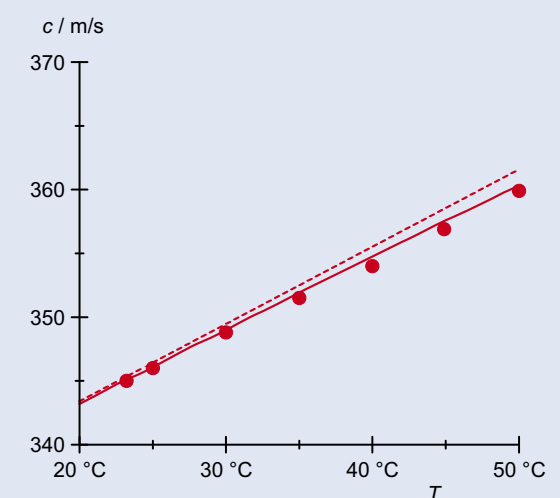
Abb. 3 Schallgeschwindigkeit c in Luft in Abhängigkeit von der Temperatur T . durchgezogene Linie: berechnet gemäß Gleichung 3, gestrichelte Linie: berechnet gemäß Gleichung 5.
