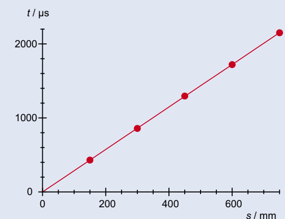
Abb. 2 Schalllaufzeit t in Luft in Abhängigkeit von der Laufstrecke s bei Raumtemperatur.
