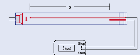
Abb. 1 Schematische Darstellung des experimentellen Aufbaus.
