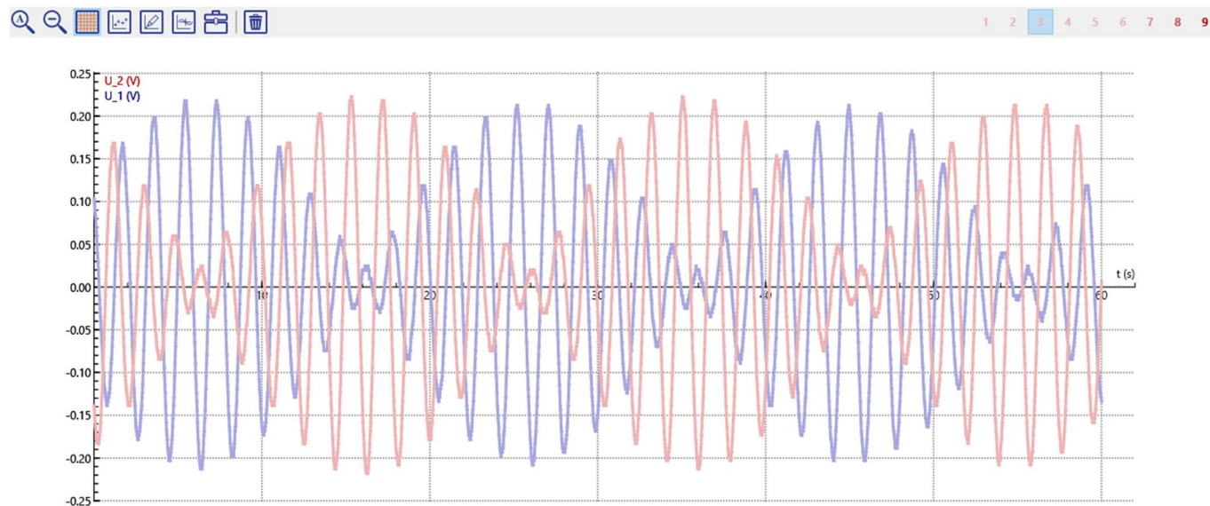
Fig. 5: Auslenkung-Zeit-Diagramm der gekoppelten Schwingung mit maximaler Schwebung
