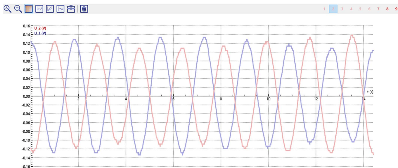
Fig. 4: Auslenkung-Zeit-Diagramm der gegenphasigen gekoppelten Schwingung
