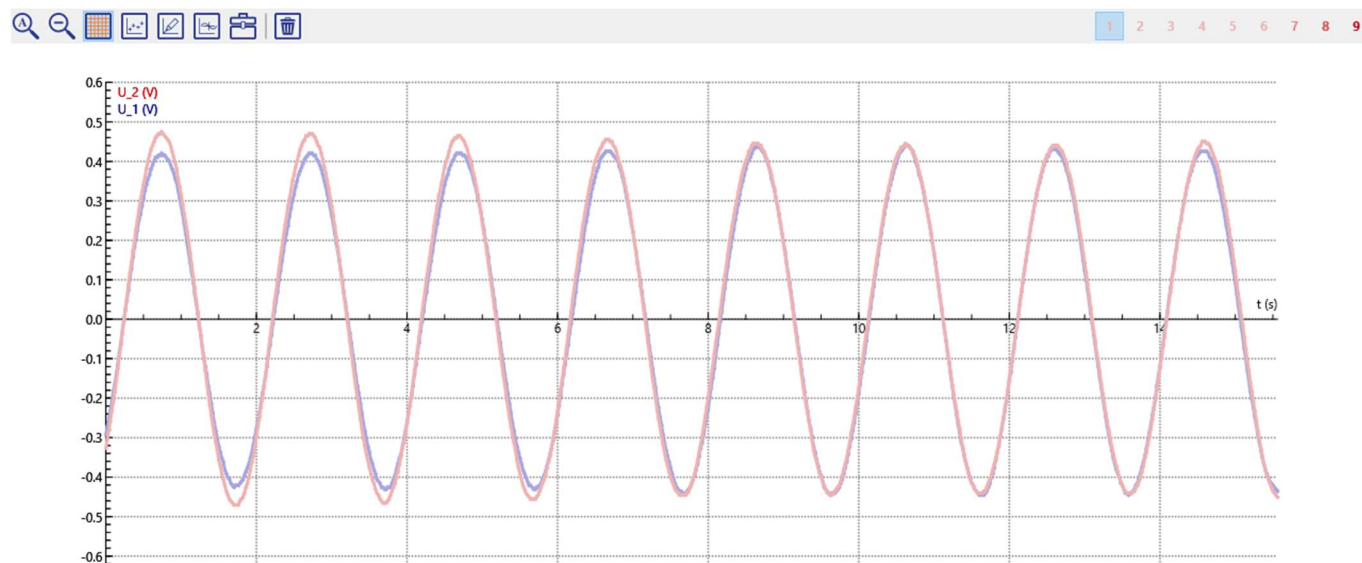
Fig. 3: Auslenkung-Zeit-Diagramm der gleichphasigen gekoppelten Schwingung
