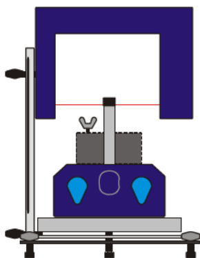
Fig. 2 Ausrichtung der Lichtschranke
