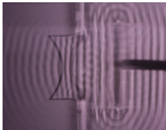
Fig. 2b: Brechung von ebenen Wellen an einer Bikonkavlinse. Die Vorderkanten der Linse sind mit Hilfe zweier langer, hochkant gestellter Quader abgeschirmt, um unerwünschte Randeffekte wie Beugungs- und Interferenzerscheinungen zu minimieren
