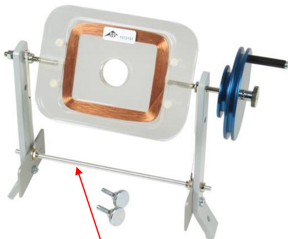
Fig. 1: Trava de transporte para a bobina plana em suporte giratório
