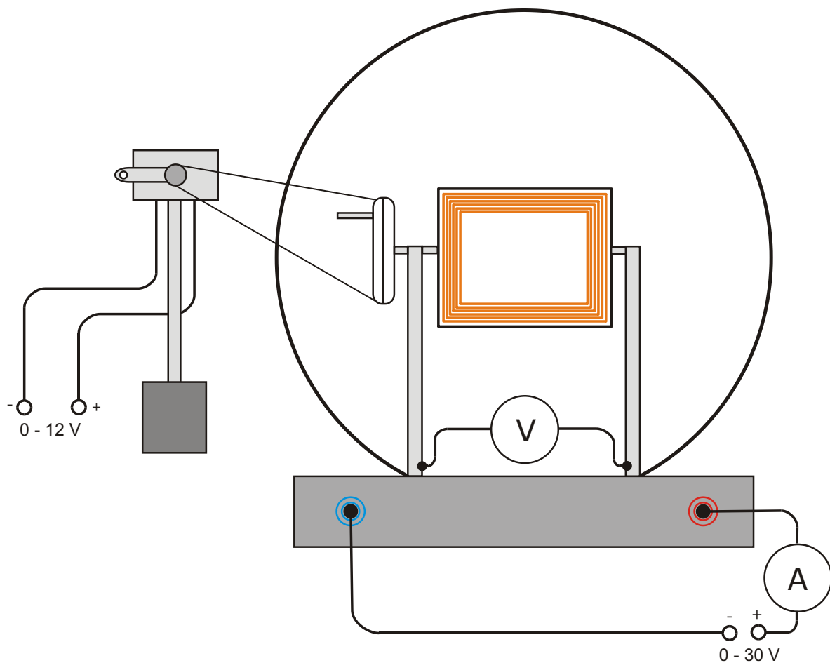
Fig. 2: Montagem da experiência com a bobina plana em suporte giratório e motor de impulso
