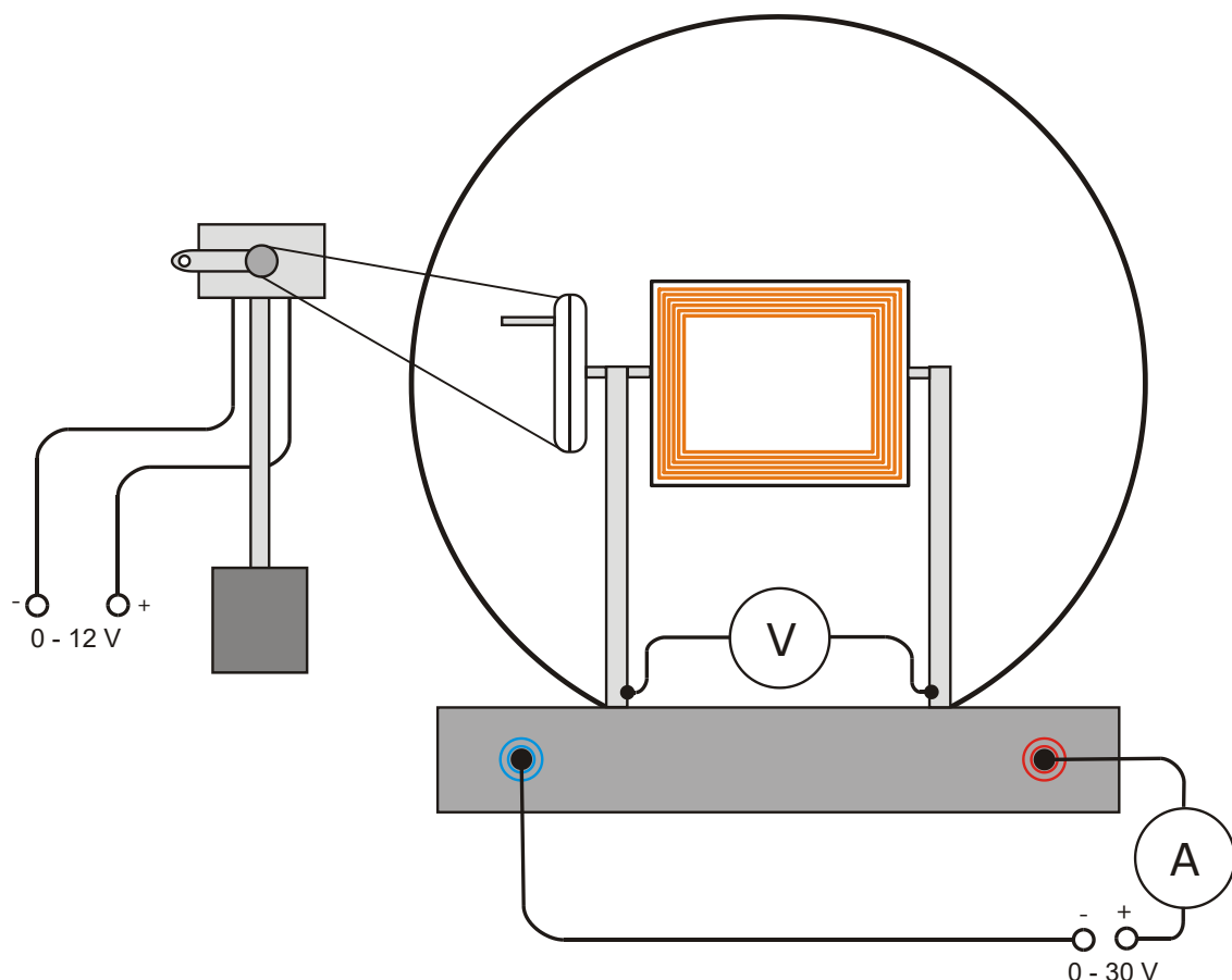
Fig. 2: Montaje experimental de la bobina plana en marco giratorio y motor de accionamiento
