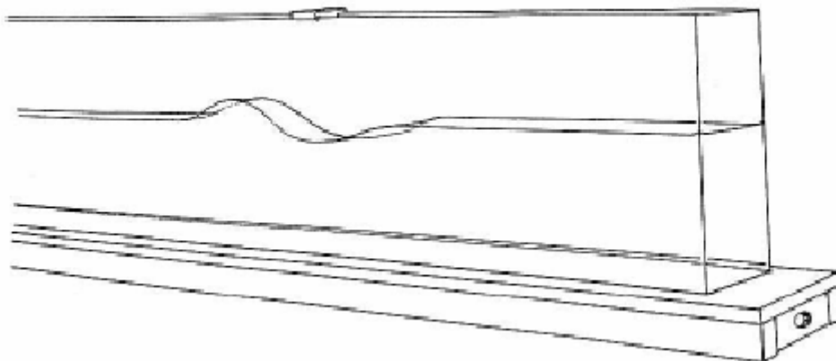
Abb. 2 Erzeugung einer nichtperiodischen Welle
