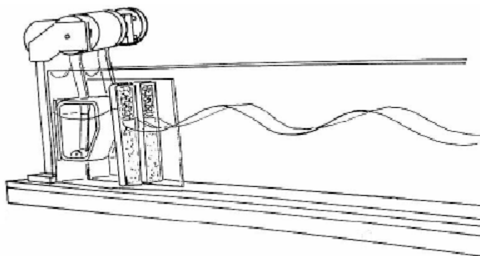
Fig. 4 Superposition déphasée des ondes
