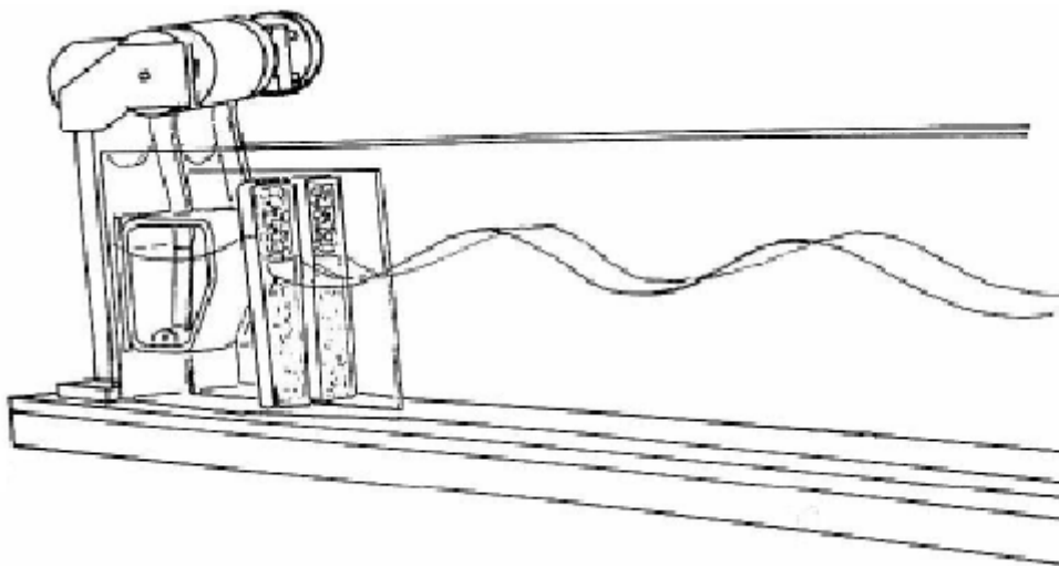
Abb. 4 Phasengleiche Überlagerung der Wellen
