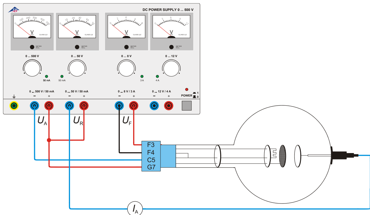
Fig. 4 Disposición de Franck-Hertz
