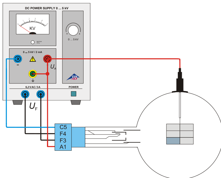
Fig. 1 Excitación por bombardeo de electrones
