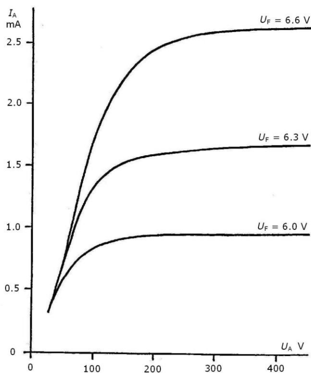
Fig. 2 Linhas características de diodo
