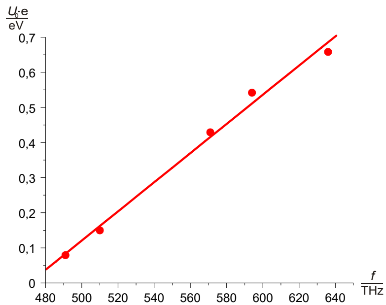
Abb.1 Grenzenenergie U_0 \cdot e in Abhängigkeit der Frequenz f
