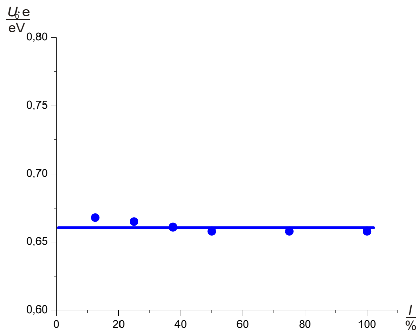
Abb. 2 Grenzspannung U_0 in Abhängigkeit der Lichtintensität I bei einer Wellenlänge von 472 nm
